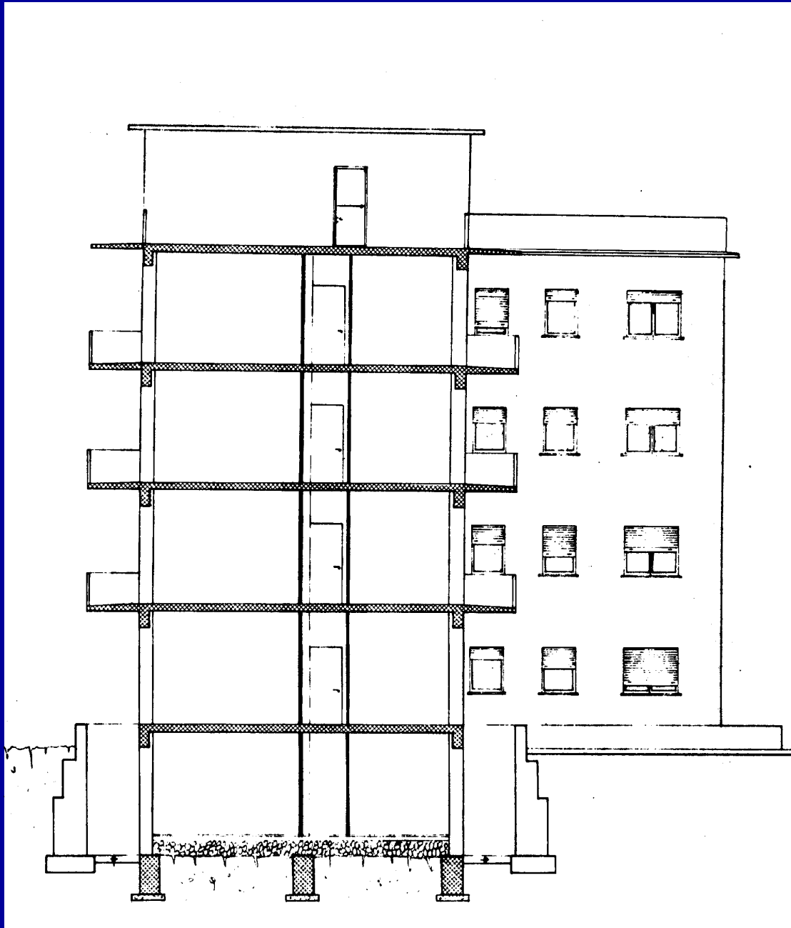
Sezione
