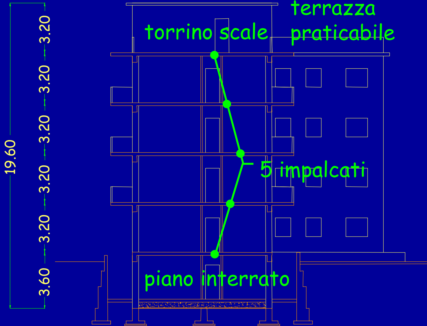
Sezione
