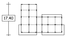
Impalcato tipo (con sbalzi)
