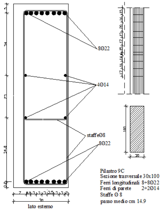
pilastro
