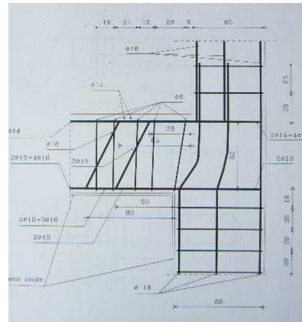
nodo trave-pilastro
