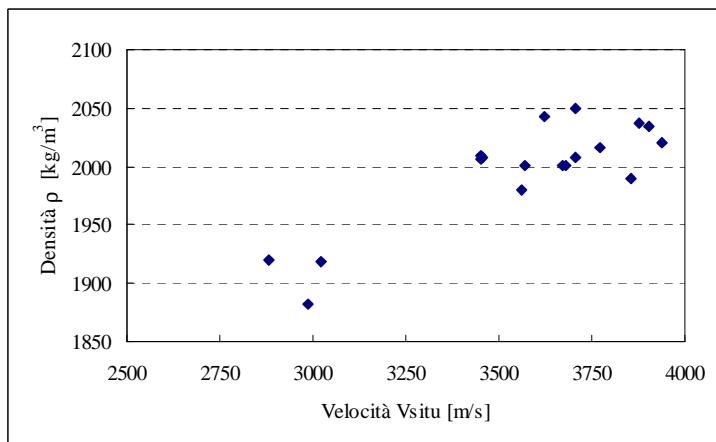
Velocità - Densità
